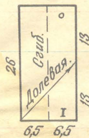
Манжета, 2 дет.
