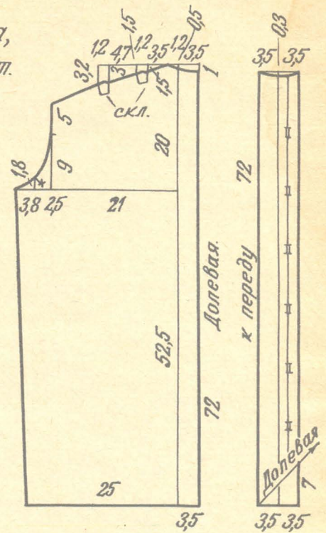
Перед, 2 дет.
